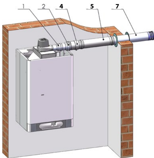
Дымоудаление 1х 100 выхлоп (горизонт.)
