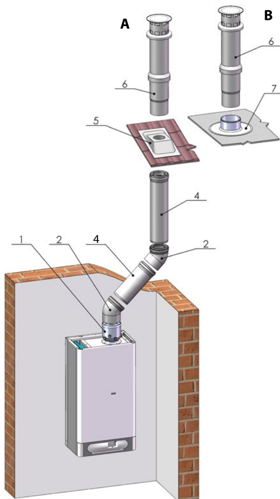
Дымоудаление \varnothing 80/125 вертик.
