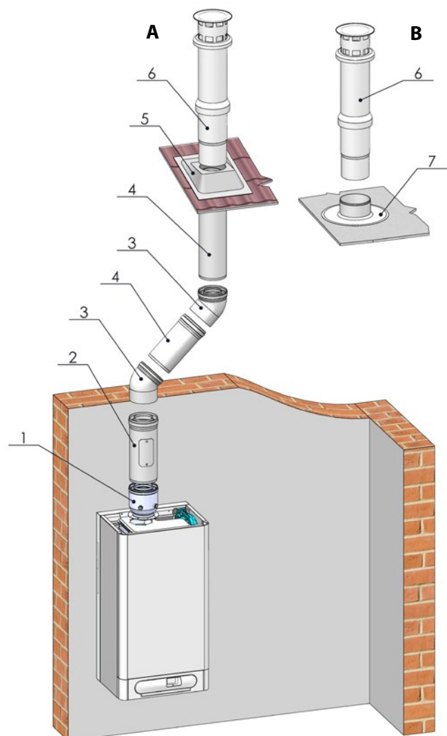
Дымоудаление \varnothing 80/125 вертикал.
