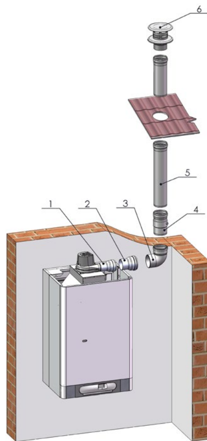
Дымоудаление 1х 100 выхлоп (вертик.)
